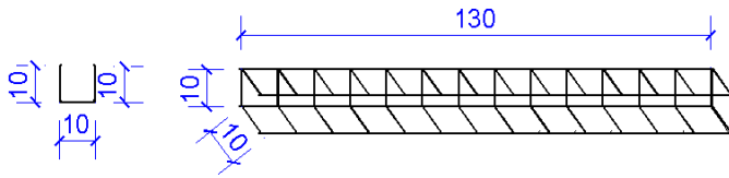
U130-30 10'lük "U" Hasır
