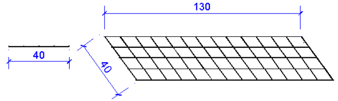
D130-40 Düz Hasır
